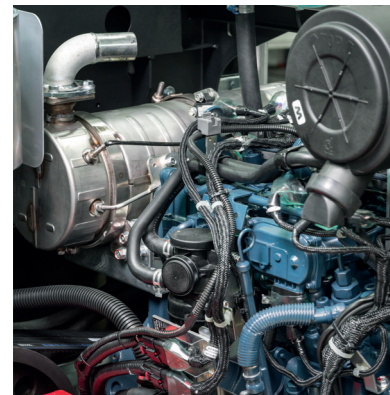
Tier 4/Stage V motor met ingebouwd roetfilter en katalysator
